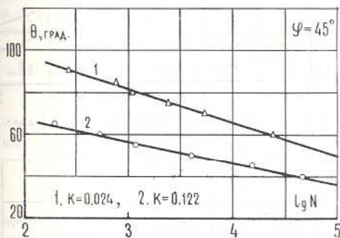
Фиг. 3. Влияние предварительного натяжения (связующее — эпокси-фенольное, частота перегиба — 95 цикл/мин).
