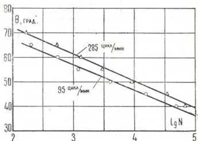
Фиг. 5. Влияние частоты перегиба.
