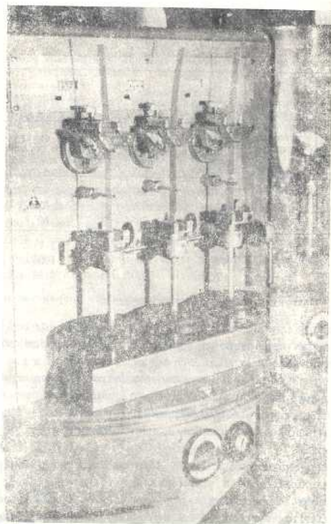
Фиг. 1. Общий вид установки для испытания материалов на циклический симметричный перегиб.
