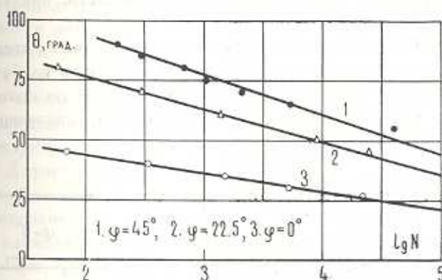
Фиг. 2. Влияние анизотропии свойства стеклошпона на деформационную выносливость при циклическом перегибе. (Связующее — эпокси-фенольное, K = 0.022 , частота перегиба — 95 цикл/мин).
